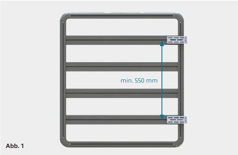
Mindestabstand zwischen den Universalhalterungen
