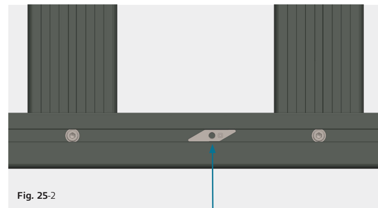
Fig. 25-2 Inserte el bloque deslizante con la marca «O» hacia abajo (flecha).
