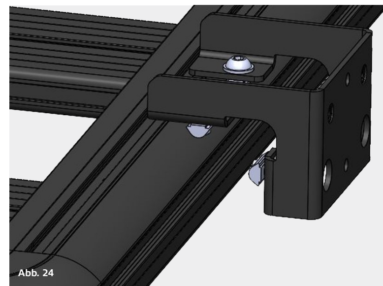
Nutensteine zum Eindrehen
