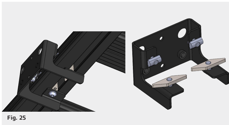
Fig. 25 Tacos deslizantes para atornillar
