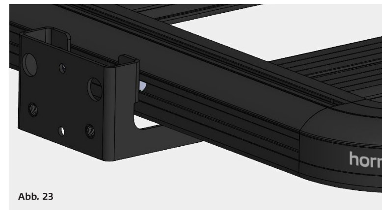
Markisenhalter unten
