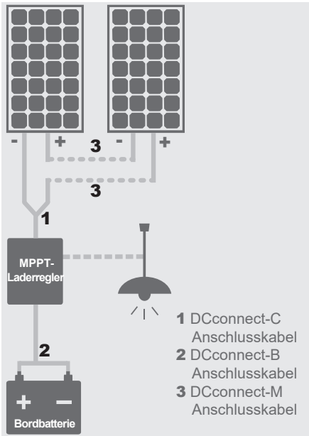
Abb. 3: Anschlussprinzip 2 Module in Reihe
