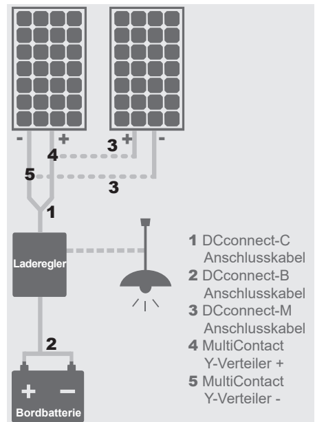
Abb. 2: Anschlussprinzip 2 Module parallel bei 12 V Modulspannung
