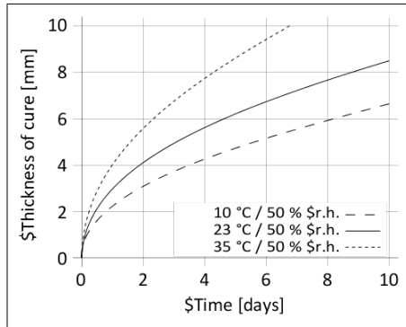
Diagramm 1: Durchhärteschwindigkeit Sikaflex®-554
