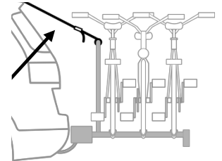
Figura 21: Cinghia di scarico trazione
