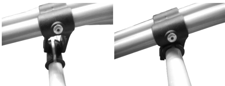
Figure 6 e 7: Posizionamento barra di espansione
