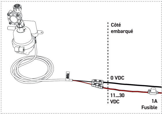
Figure 15 : Raccordements électriques
