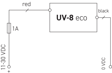
Figure 14 : Plan de Raccordements électriques
