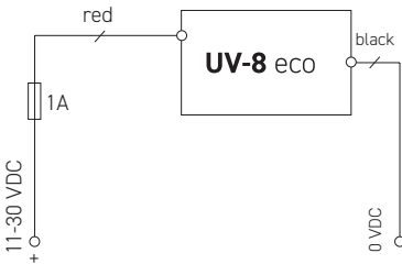
Abbildung 16: Elektrischer Anschluss
